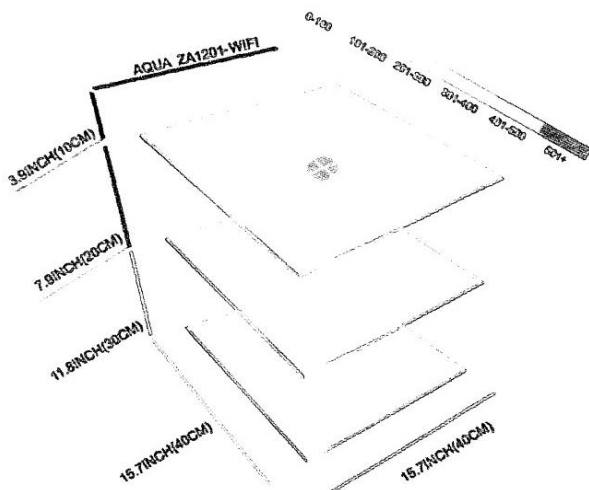
PAR measurement of a 40X40X40cm tank
